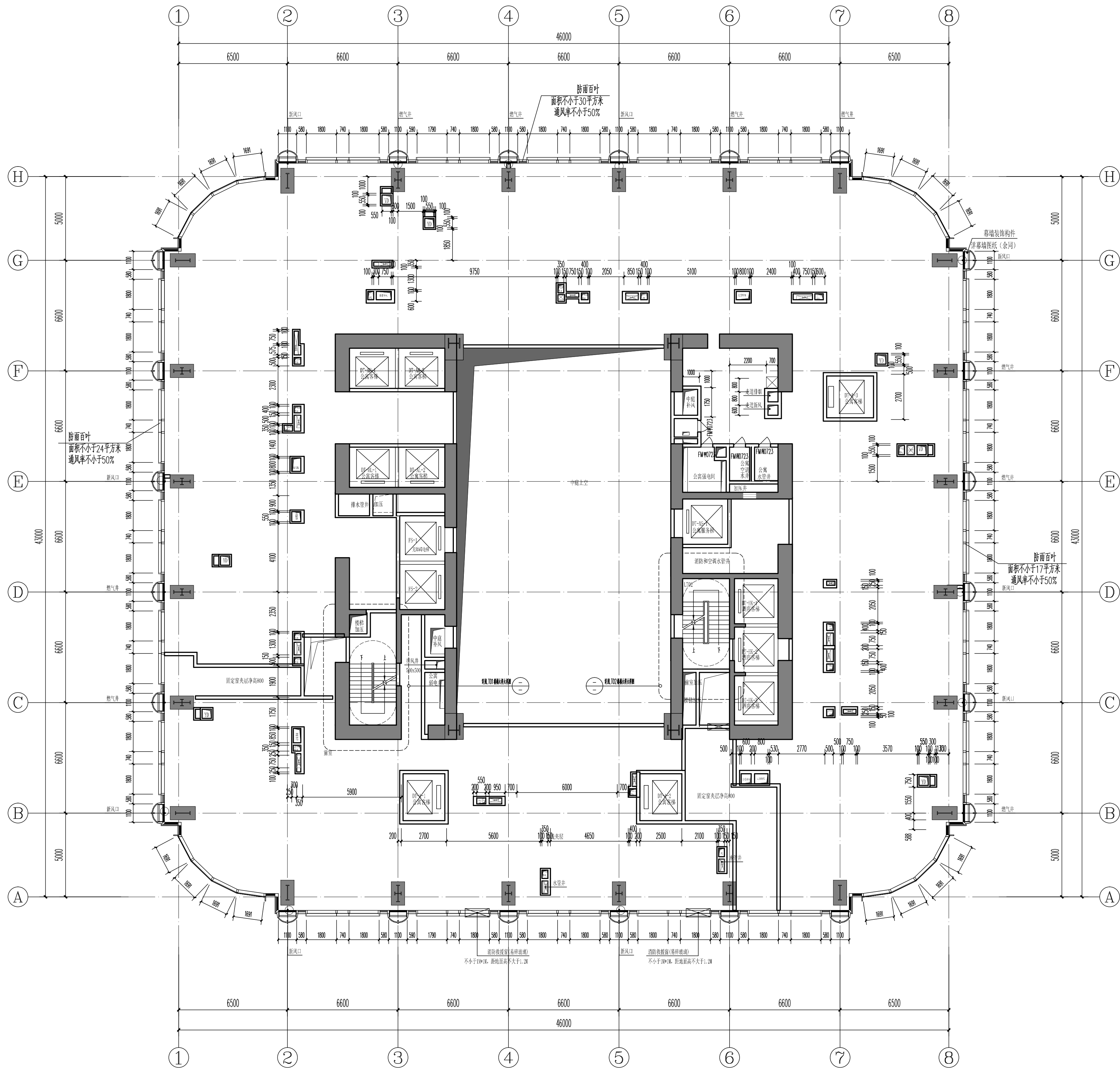
二十六夹层平面图 1:150
